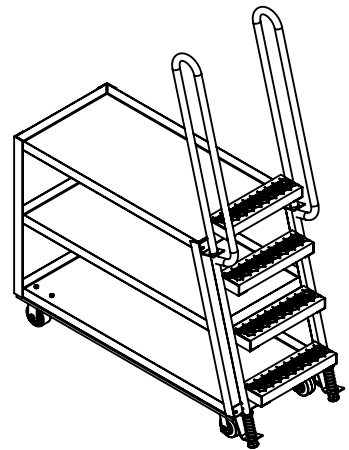
ISOMETRIC VIEW SCALE: 1:32
