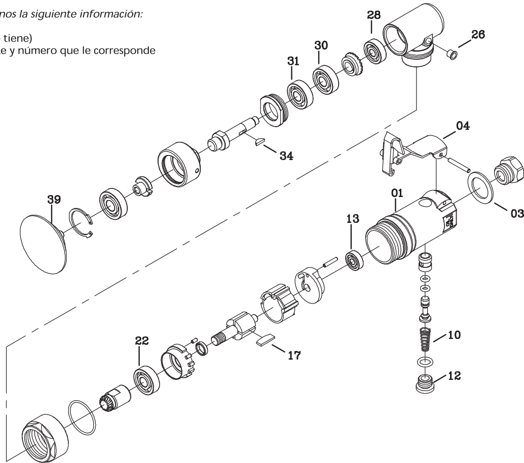
Figura 3 - Ilustración de las Partes de Repuesto
