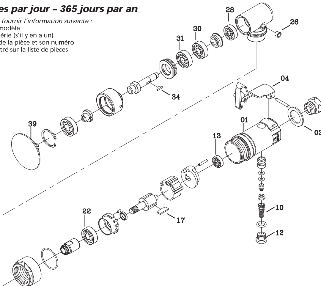
Figure 3 - Illustration des pièces de remplacement
