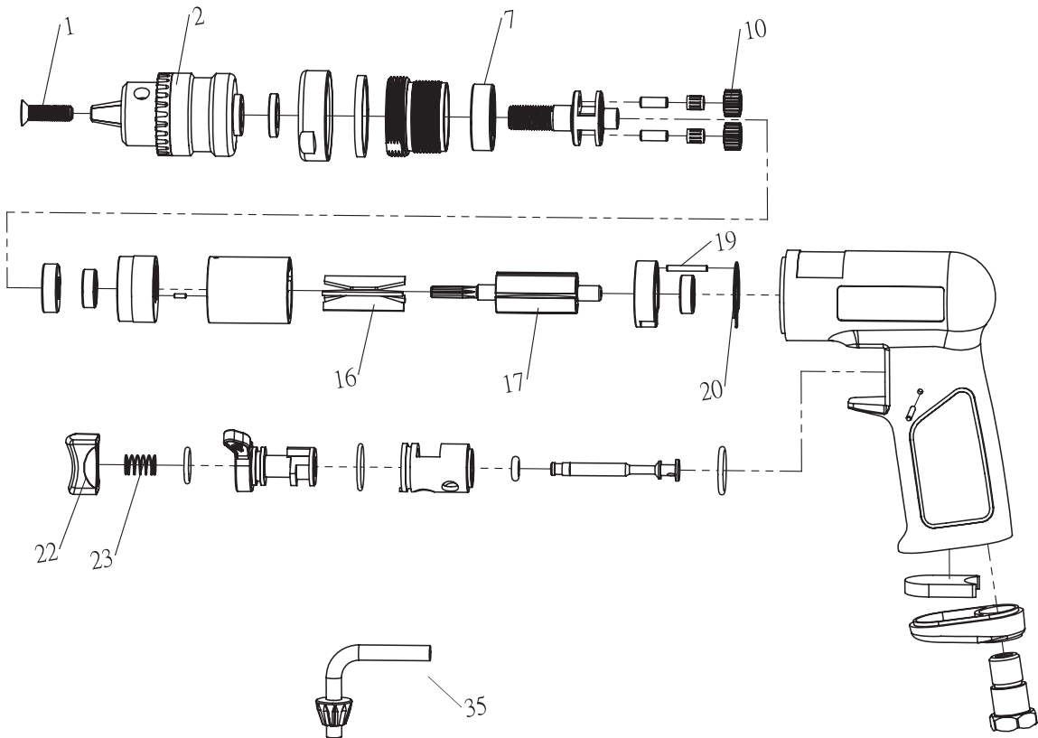
Figure 3 - Illustration des pièces de remplacement
