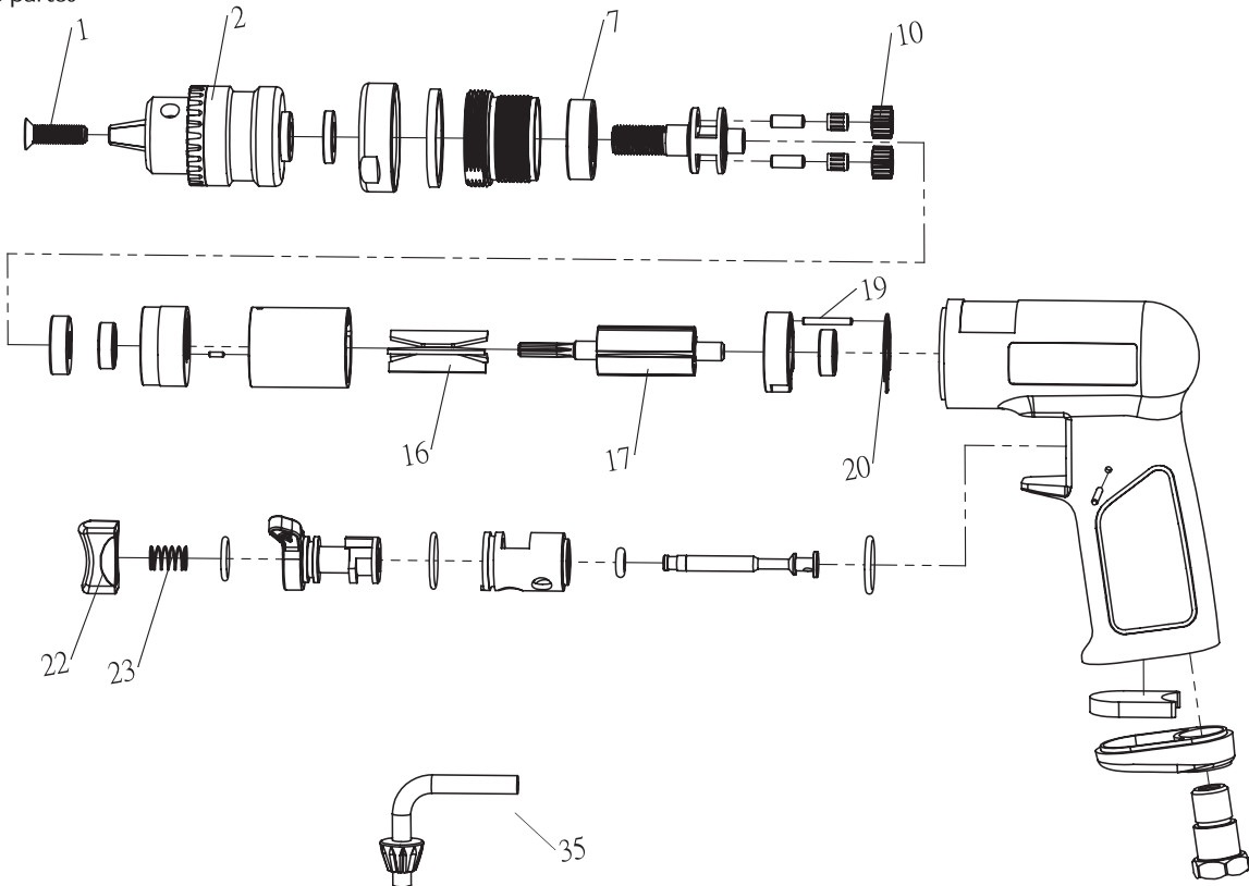
Figura 3 - Ilustración de las Partes de Repuesto
