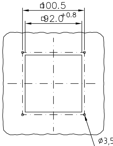
Montageausschnitt SK 3321 100/107 SK 3321 115/117 SK 3321 024/027 SK 3321 047/048 SK 3321 600/615 SK 3321 200/207 SK 3321 260
