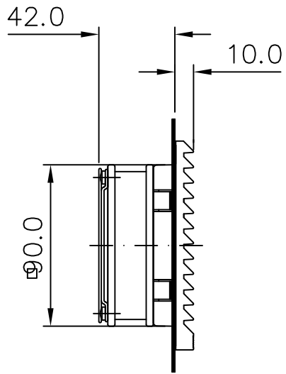
Filterluefter SK 3321 100/107 SK 3321 115/117 SK 3321 024/027 SK 3321 047/048 SK 3321 600/615
