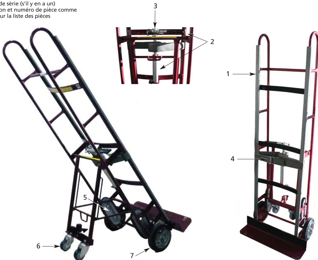
Figure 3 – Illustration des pièces détachées pour les chariots pour distributeurs automatiques
