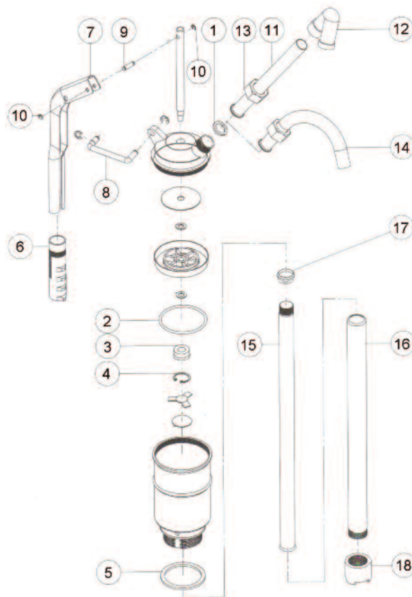
DIBUJO 2 – Ilustración de las Partes de Reparación para la Bomba de Alta Viscosidad Accionada por Palanca
