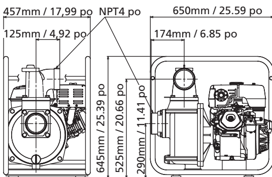
Dimensions du modèle 11G236
