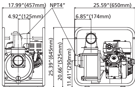
Dimensiones para el Modelo 11G236
