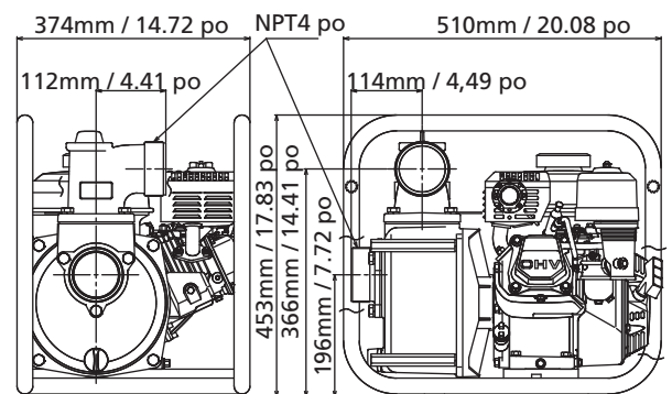
Dimensions du modèle 11G235
