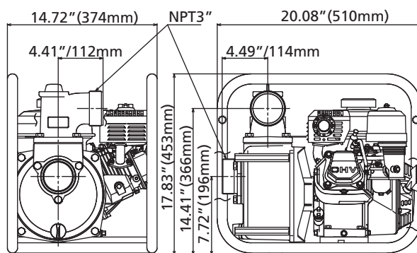
Dimensiones para el Modelo 11G235
