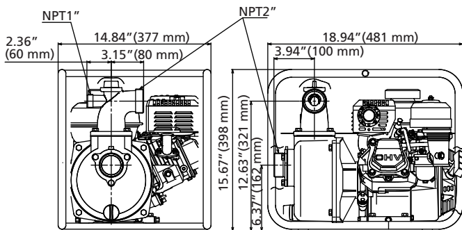
Dimensiones para el Modelo 11G227
