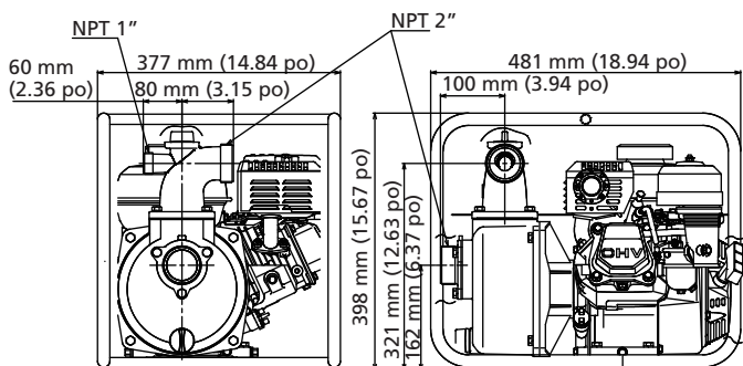
Dimensiones para el Modelo 11G227
