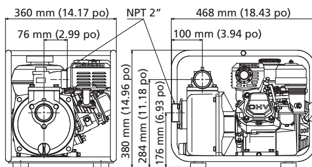
Dimensions du modèle 11G228
