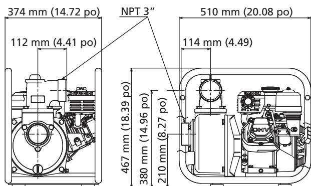
Dimensions du modèle 11G229
