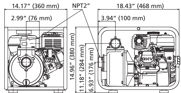
Dimensiones para el Modelo 11G228
