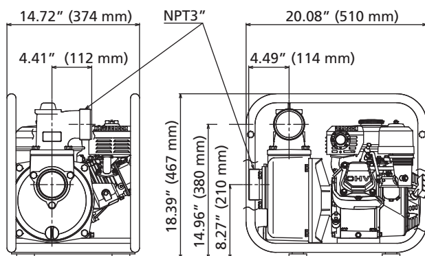
Dimensiones para el Modelo 11G229
