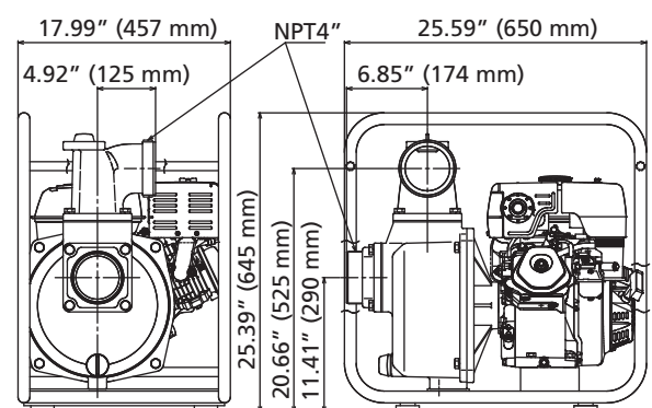
Dimensiones para el Modelo 11G230
