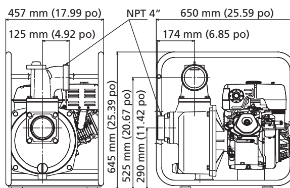
Dimensions du modèle 11G230
