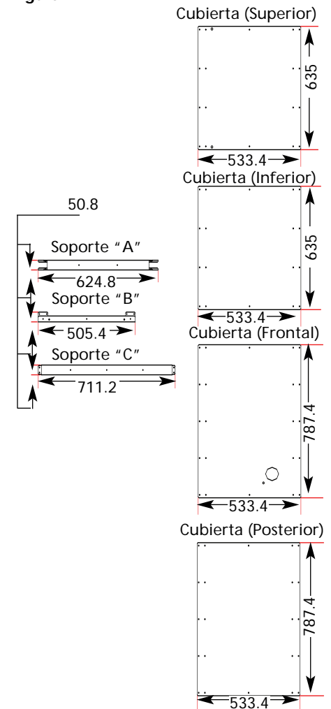
Figura 3 - Dimensiones de las Cubiertas y Soportes
