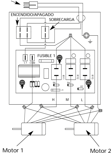
Figura 4 - Diagrama de Circuitos Eléctricos
