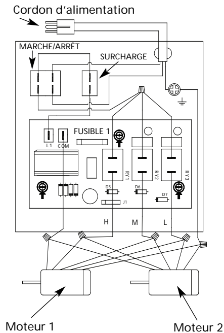
Figure 4 – Schéma du circuit électrique
