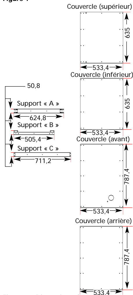
Figure 3 - Dimensions des couvercles et des supports
