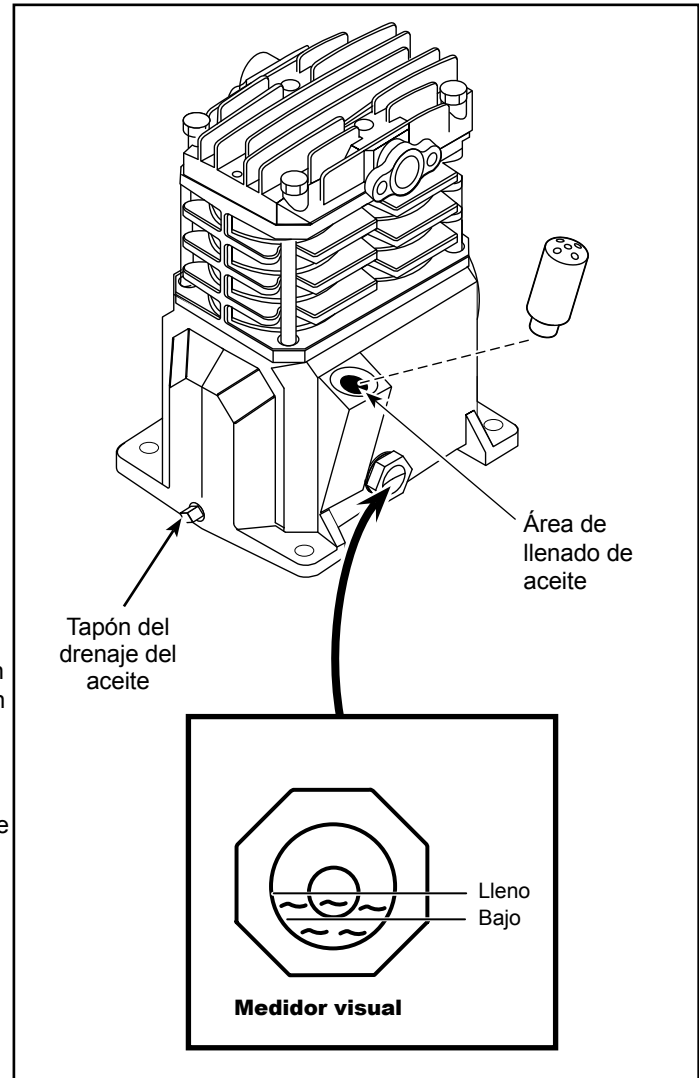
Figura 5 - Lubricacion
