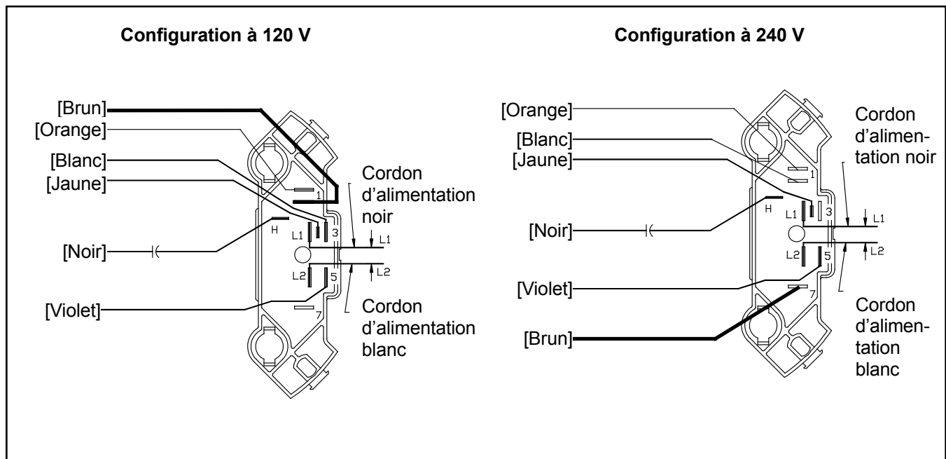
Figure 4 - Configuration 120 V et 240
