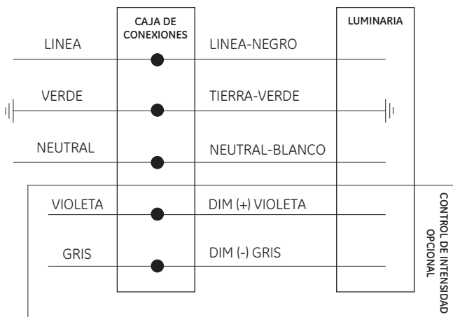
CABLEADO DE SUMINISTRO
