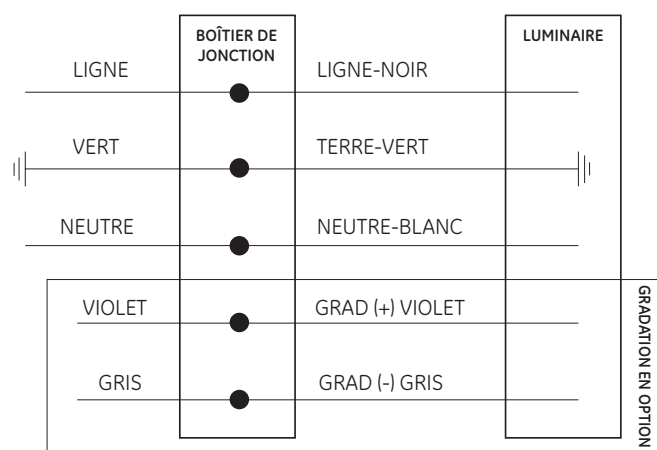
CÂBLAGE D'ALIMENTATION
