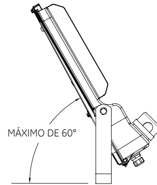
FIGURA 5. Alcance máximo de puntería con PE
