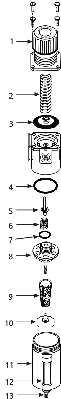
Figure 6 – Illustration des pièces détachées pour le filtre/régulateur
