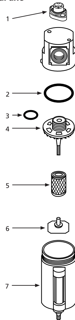
Figura 4 – Ilustración de las Partes de Reparación del Filtro Coalescente
