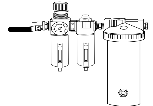
Figura 1 SECADOR DESECANTE
