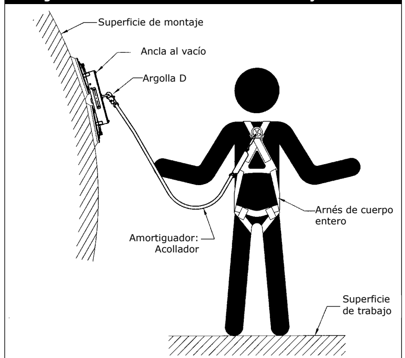
Figura 7: Uso del sistema autónomo de anclaje al vacío
