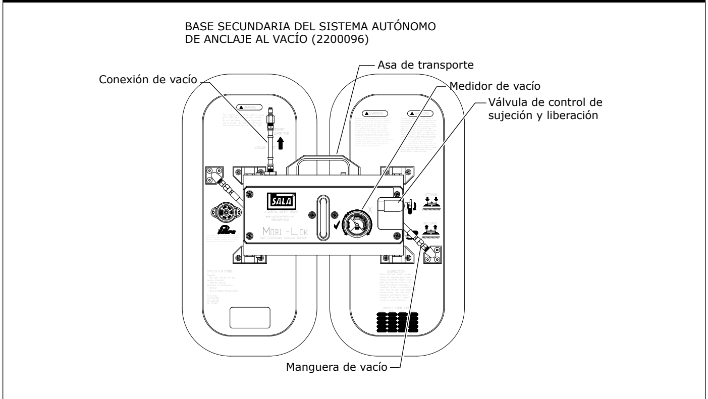
Figura 6 continuación - Identificación de componentes - sistema autónomo de anclaje al vacío Mobi-Lok
