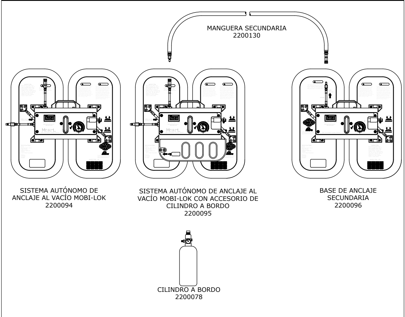
Figura 1 - Sistema autónomo de anclaje al vacío
