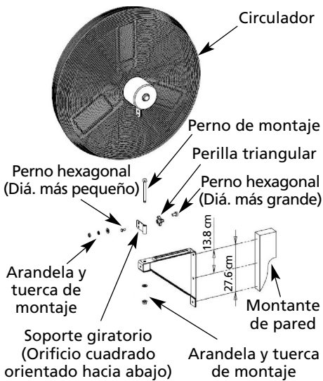
Figura 3 – Conjunto Montado en Pared
