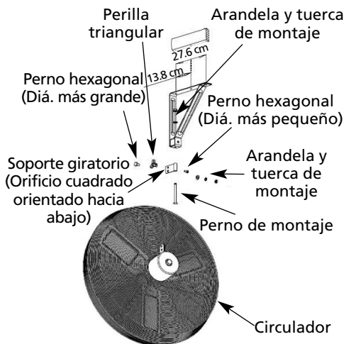
Figura 4 – Conjunto Montado en Techo
