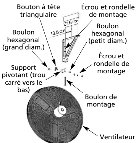
Figure 4 – Montage sur plafond
