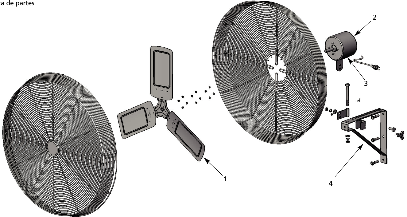
Figura 5 – Ilustración de las Partes de Reparación para los Circuladores de Aire para Uso Comercial
