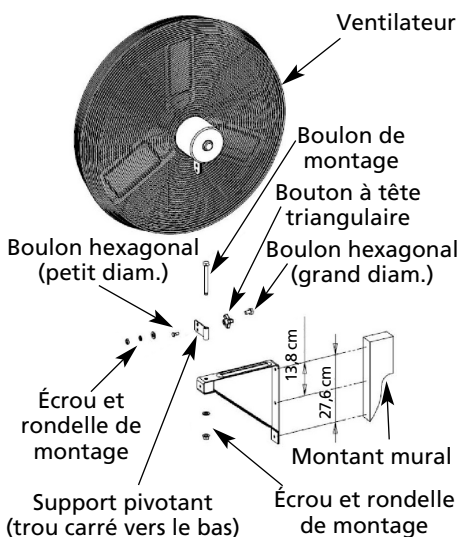
Figure 3 – Montage sur un mur
