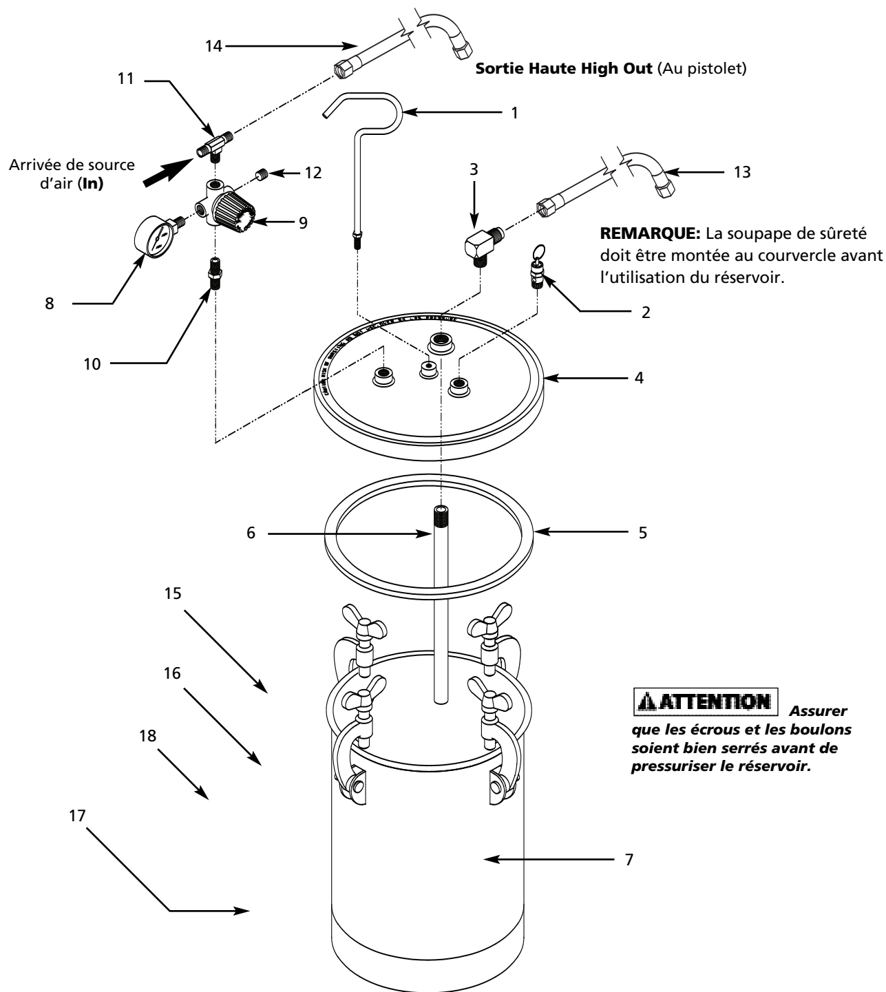
Figure 7 — Illustration de Pièces Detachées
