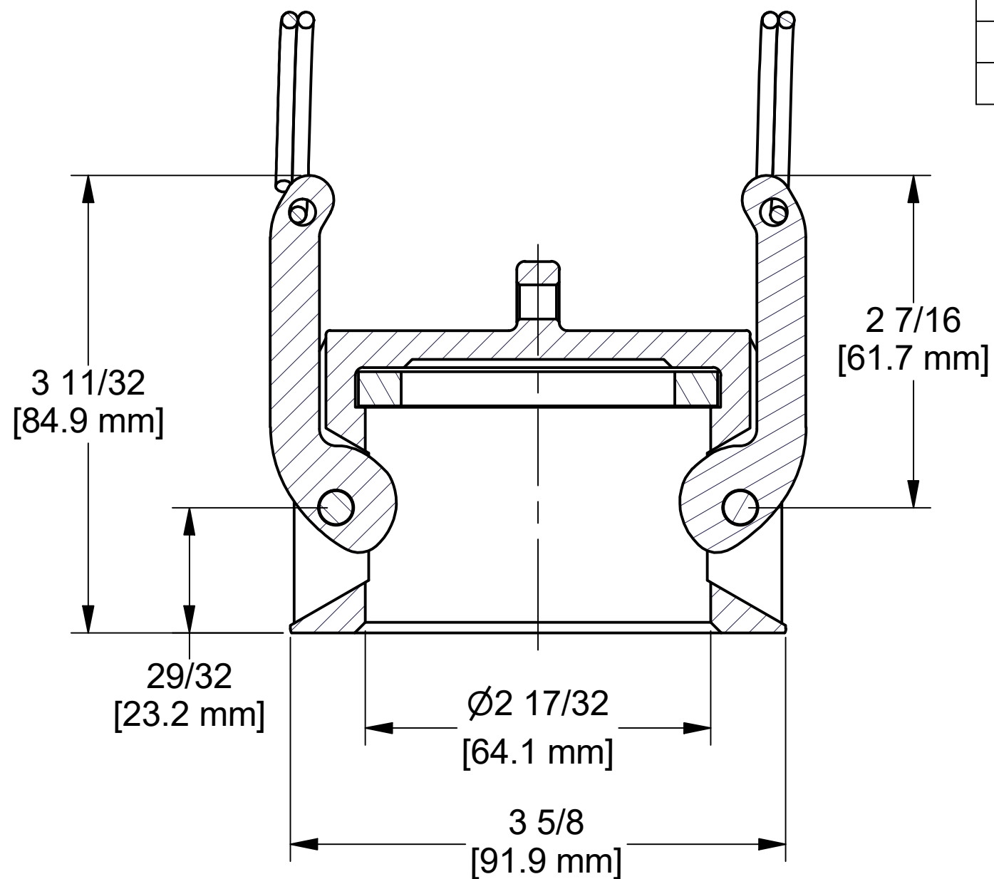
SECTION D-D SCALE 1 : 1
